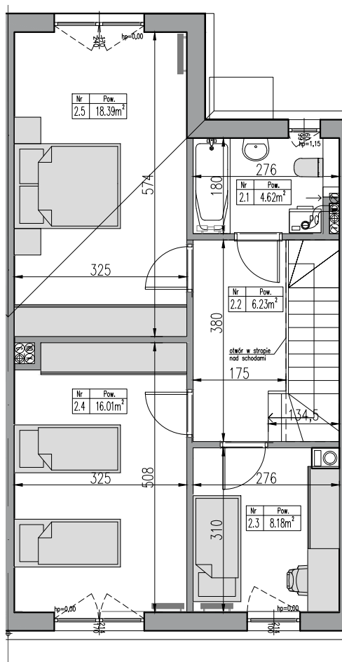
PIĘTRO
